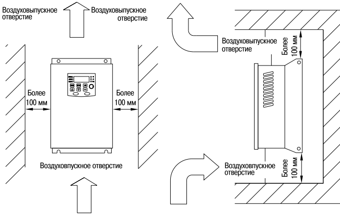
Рисунок 7 — Способ установки преобразователя частоты
