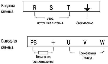
Рисунок 10 — Схема подключения силовой цепи 2 преобразователей частоты А310
