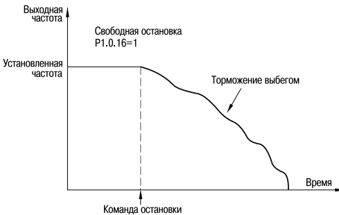
Рисунок 57 — Остановка замедлением
