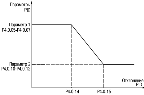
Рисунок 41 — Переключение ПИД
