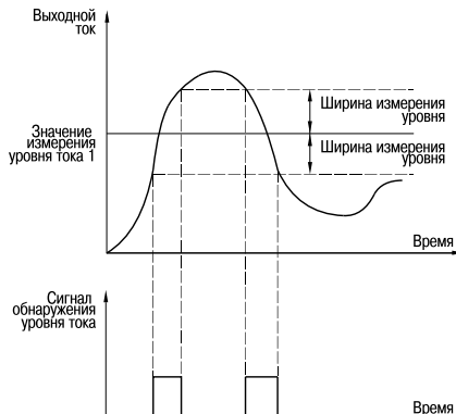
Рисунок 40 — Измерение уровня тока
