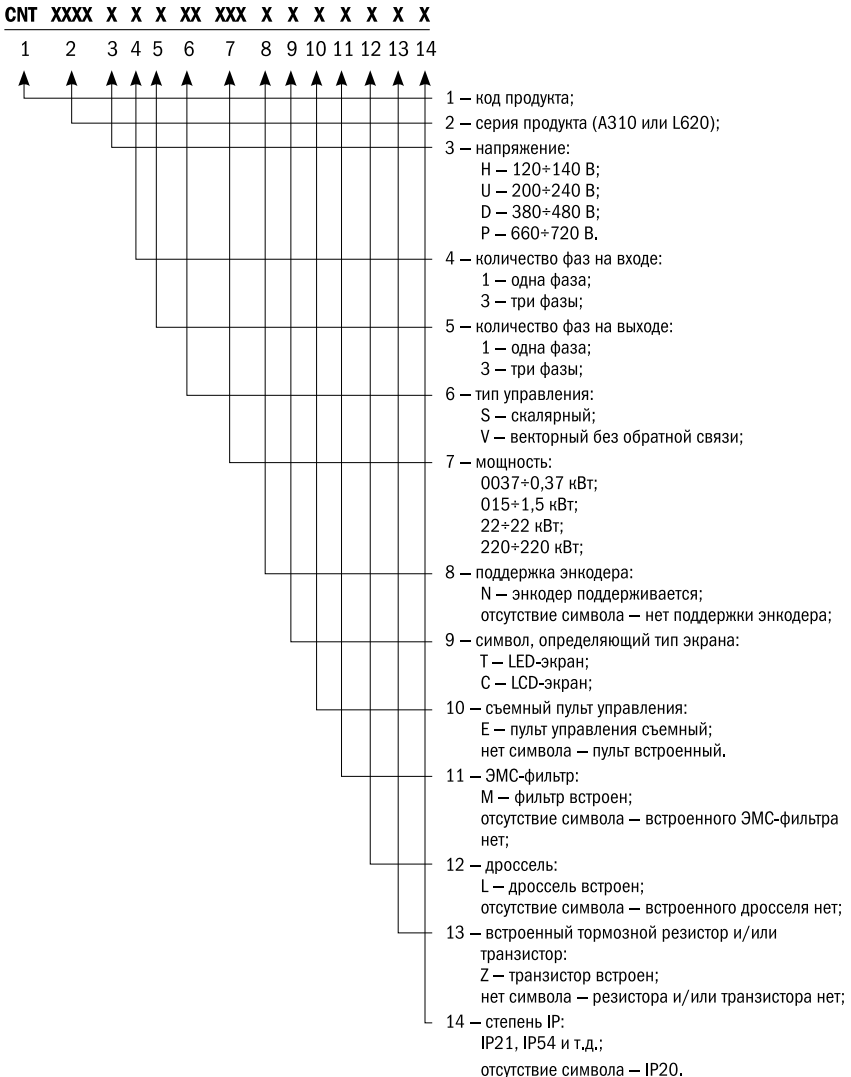
Рисунок 1 – Пример расшифровки артикула преобразователя частоты
