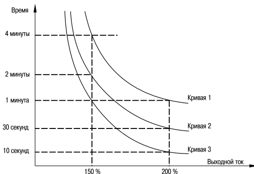
Рисунок 32 — Кривые защиты от перегрузки
