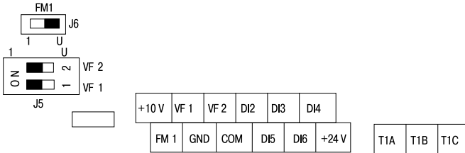
Рисунок 13 — Клеммная колодка преобразователя частоты
