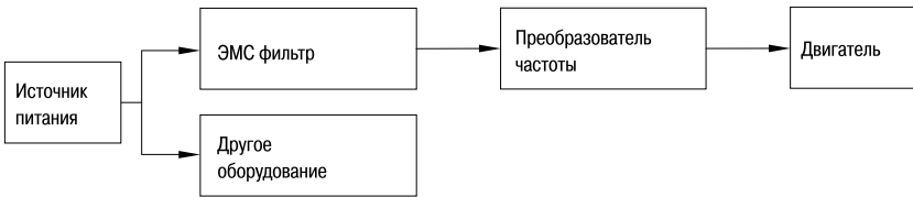
Рисунок 12 — Подключение фильтра со стороны входа
