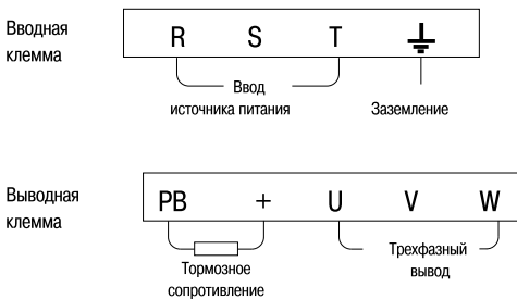
Рисунок 9 – Схема подключения силовой цепи 1 преобразователей частоты А310
