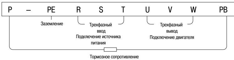
Рисунок 11 — Схема подключения силовой цепи 3 и 4 преобразователей частоты А310
